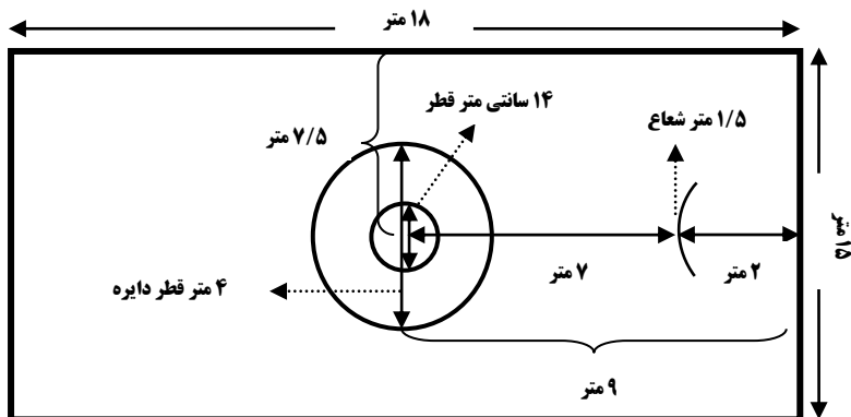
شکل شماره ۱: ابعاد زمین بازی هفت سنگ
